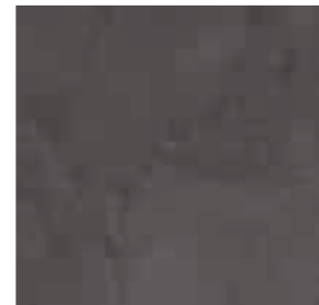
c Fog
